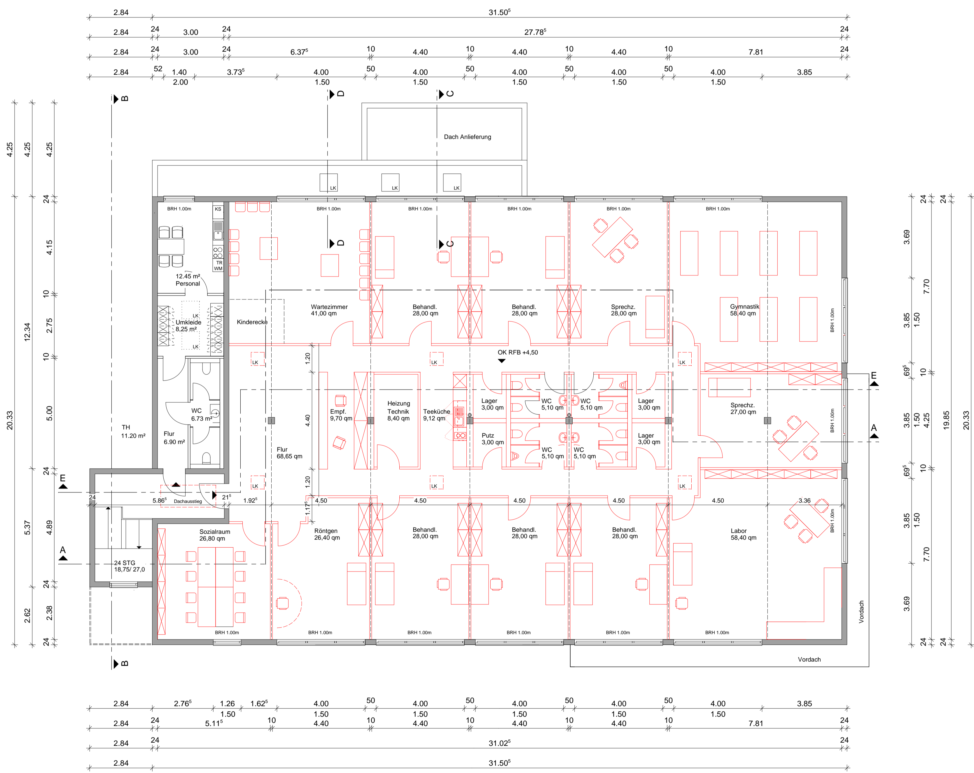
1. Obergeschoss
