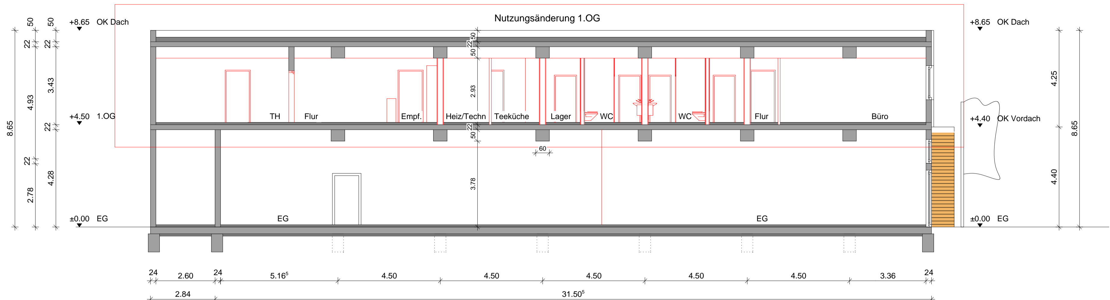
SCHNITT E - E
