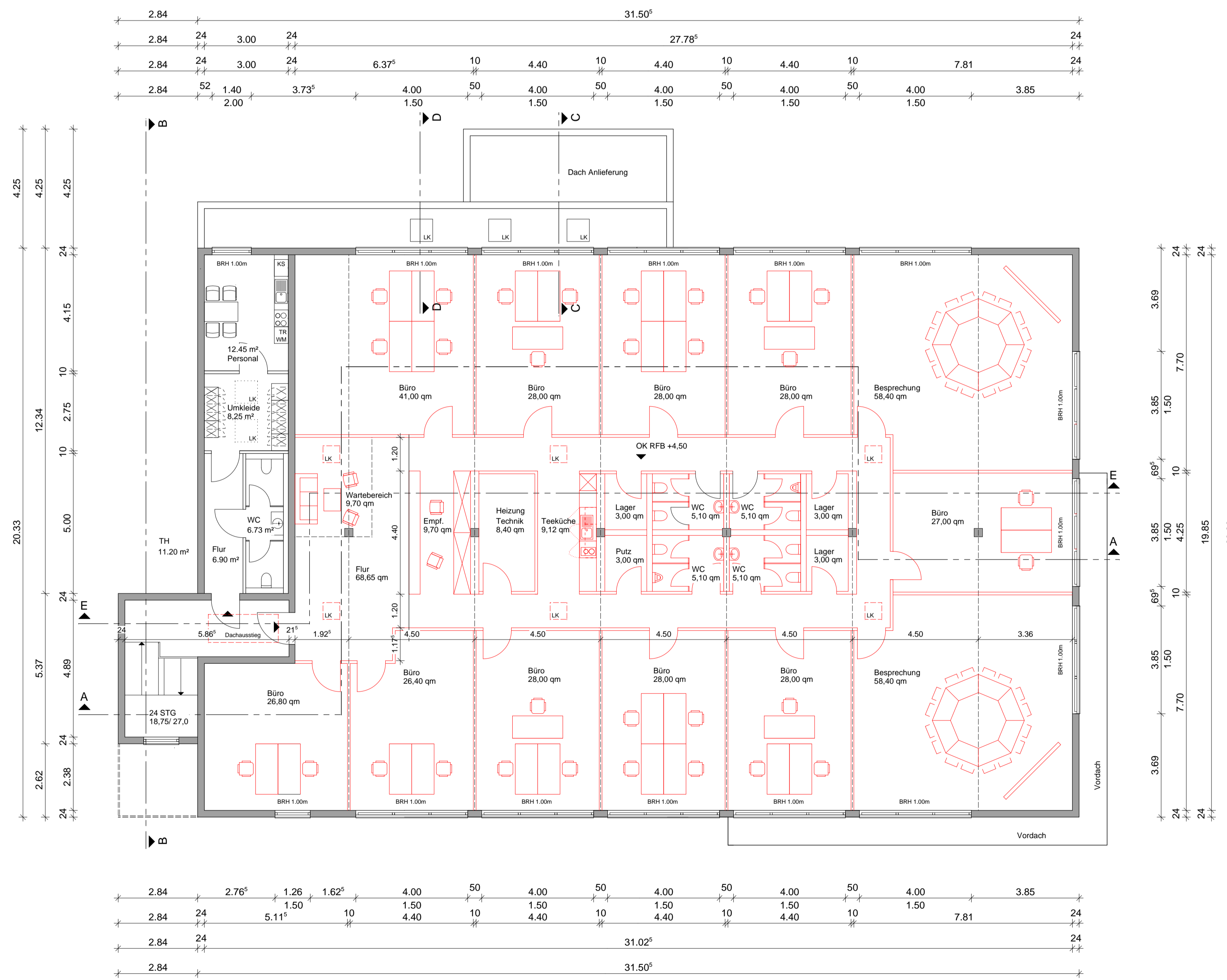
1. Obergeschoss
